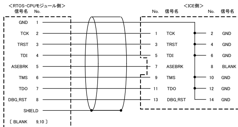
内部接続図
