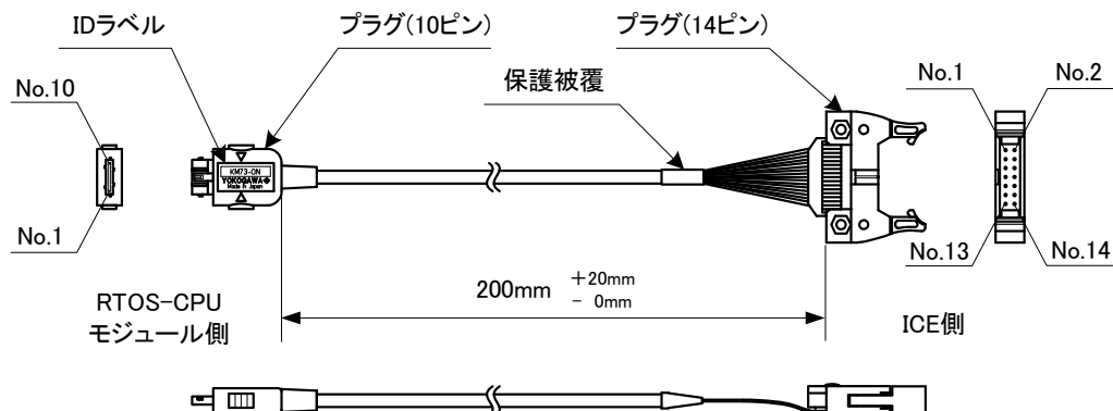
外形図
