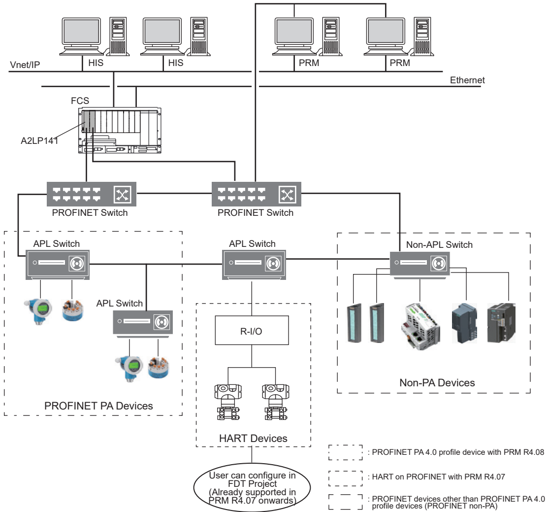
図 PROFINET 通信
